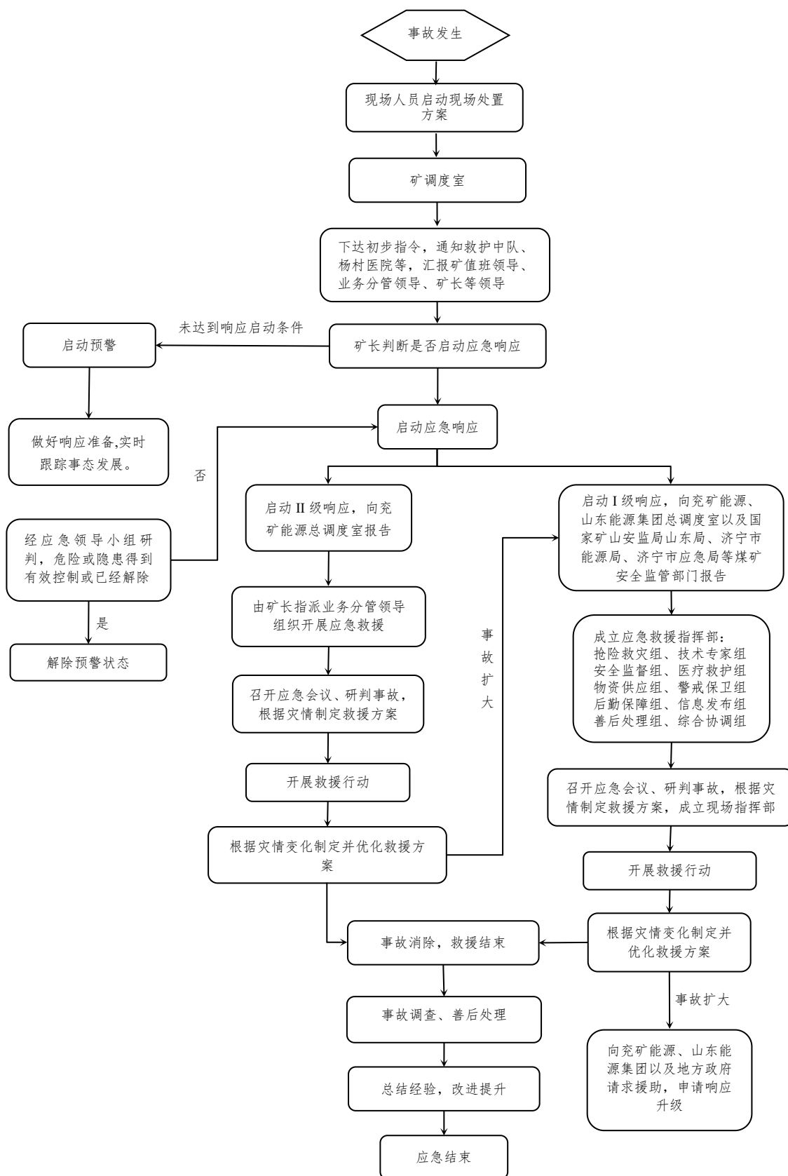
杨村煤矿应急响应流程图
